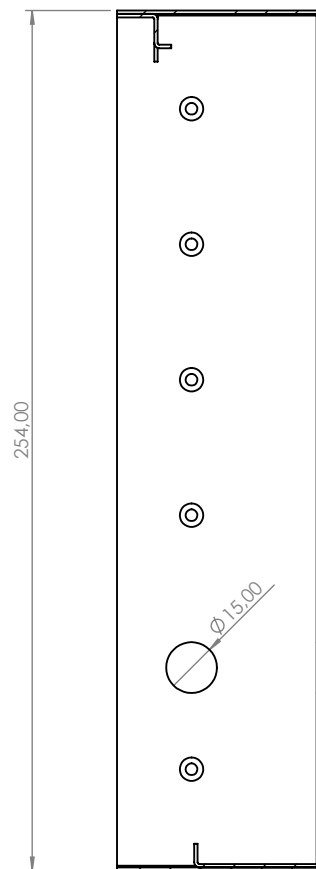
COUPE A-A
